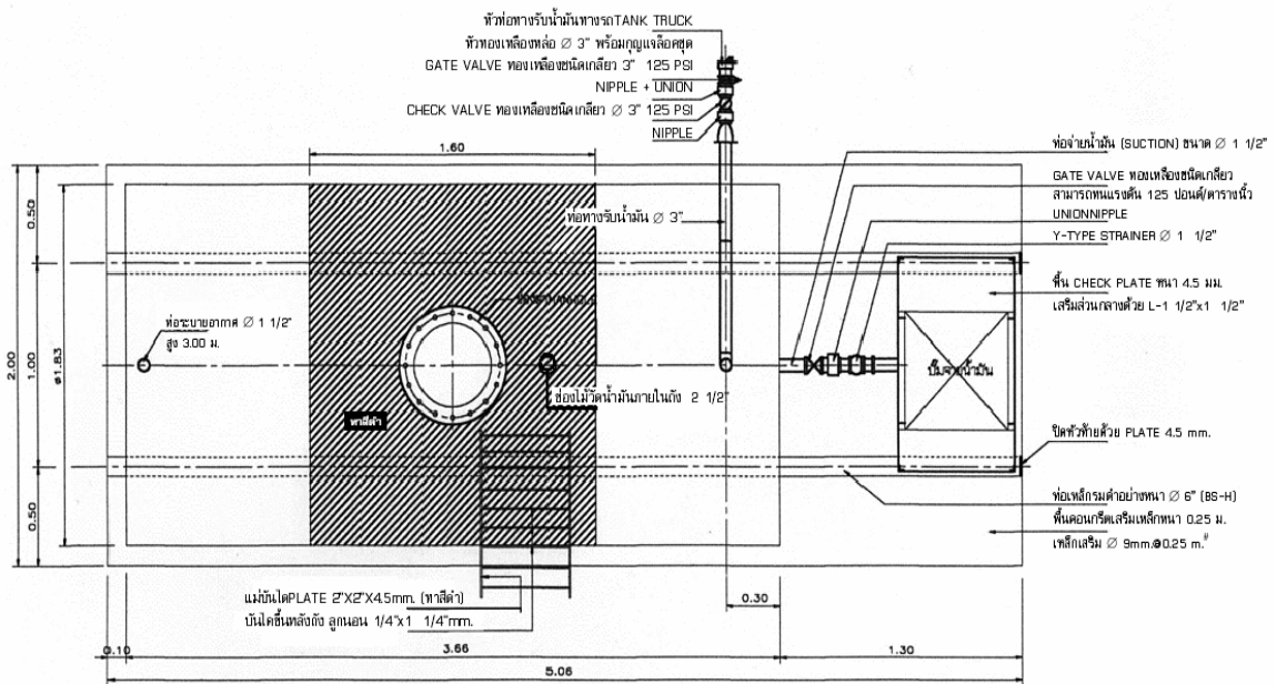
รูปที่ 4-4 แปลนถังน้ำมันฐานสกีขนาดบรรจุไม่เกิน 9,600 ลิตร
